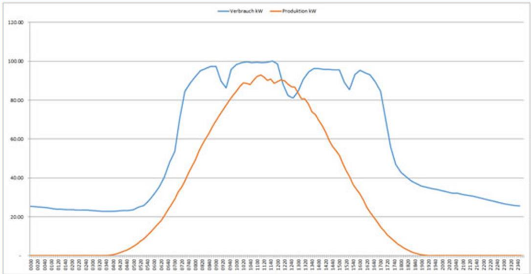
Typischer Lastgang und Solarstrom-Produktion im Tagesverlauf
